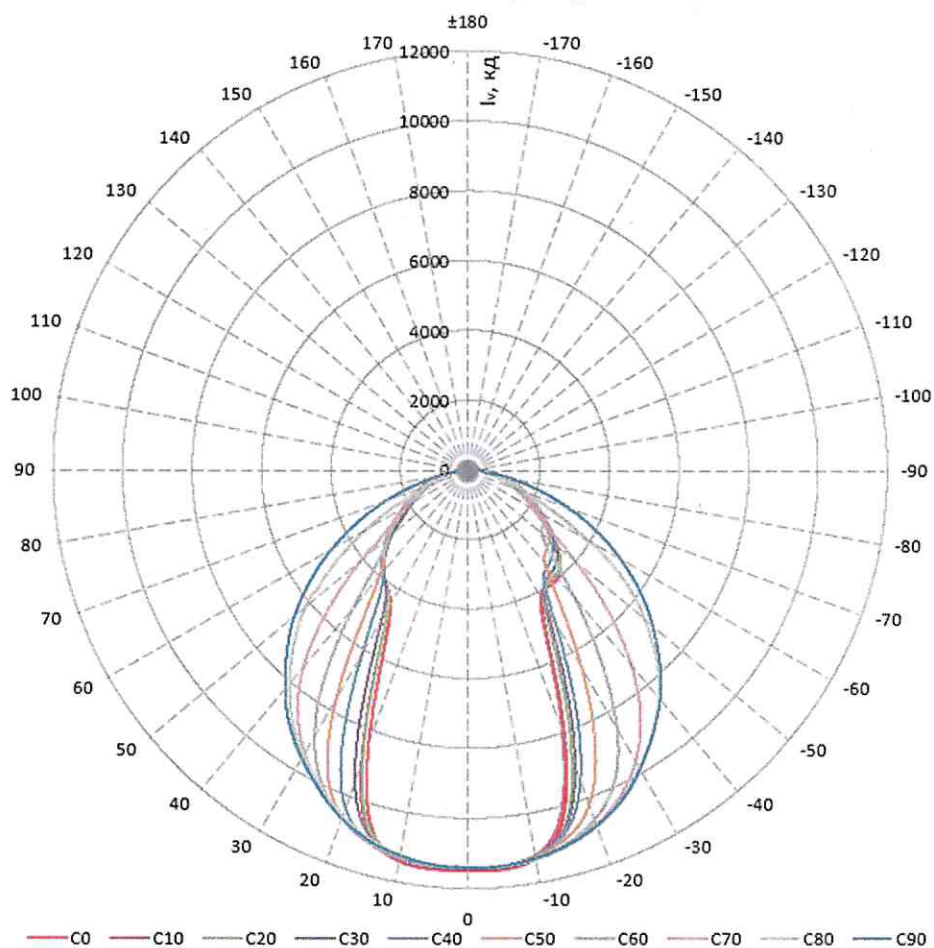
Рисунок 1. Полярные координаты
