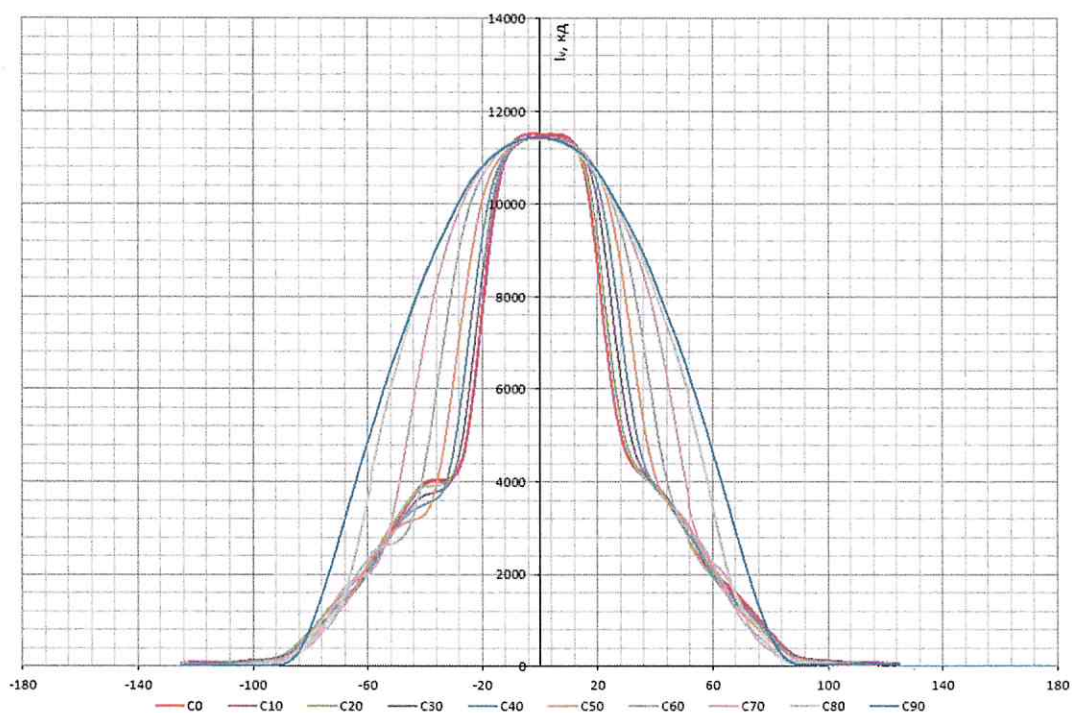
Рисунок 2. Декартовы координаты
