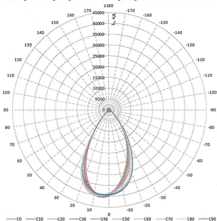
Рисунок 1. Полярные координаты
