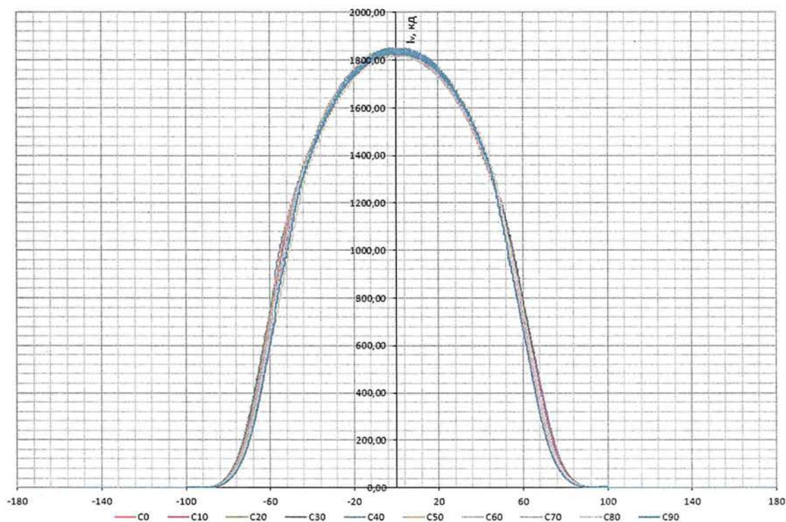
Рисунок 2. Декартовы координаты
