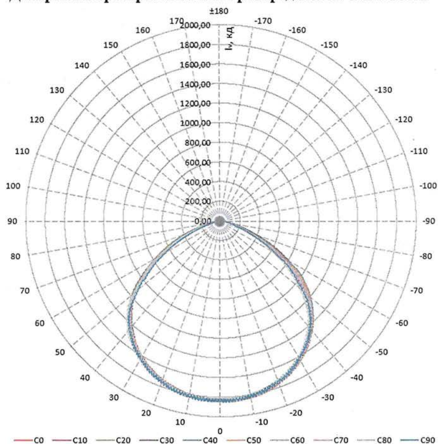
Рисунок 1. Полярные координаты
