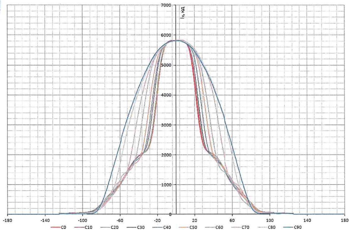
Рисунок 2. Декартовы координаты
