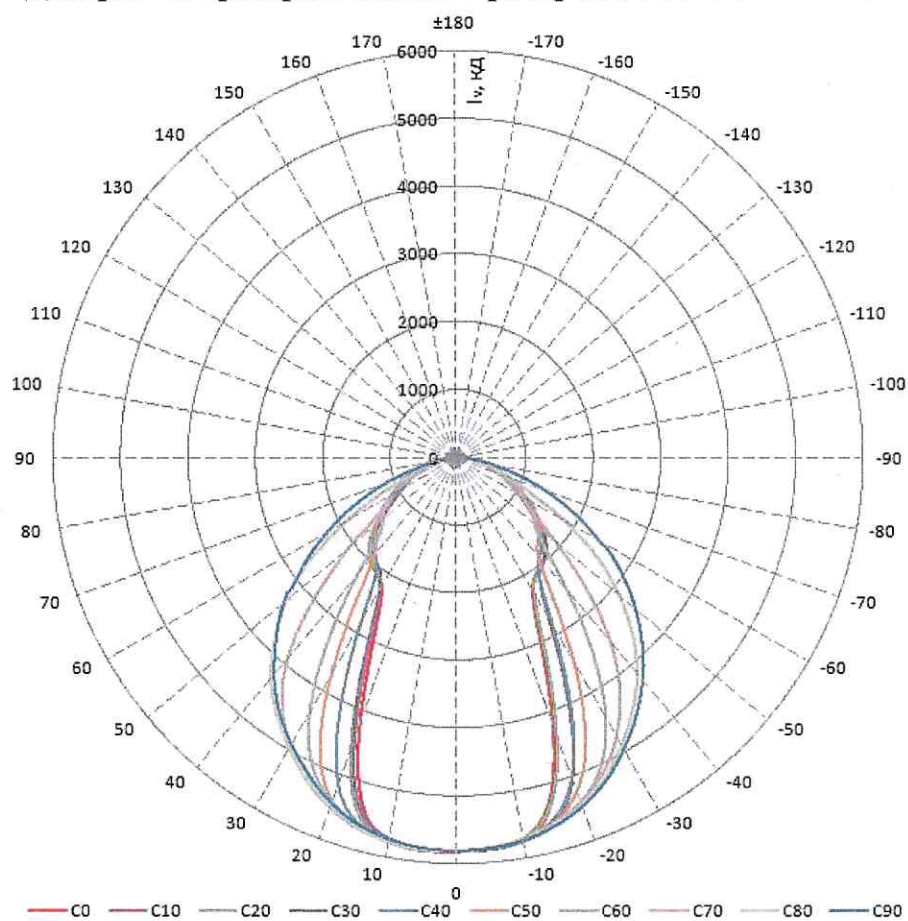
Рисунок 1. Полярные координаты
