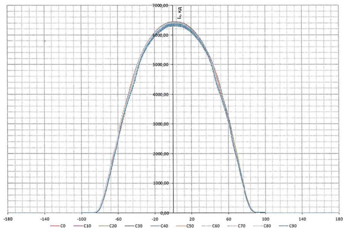
Рисунок 2. Декартовы координаты
